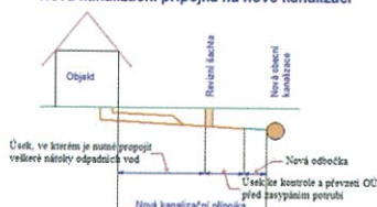
Nová kanalizační přípojka na nové kanalizaci
