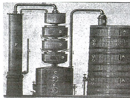
Destilační zařízení hospodářského lihovaru, A vařič, B dóm, C lutrová kolona, D efektor, F chladič
